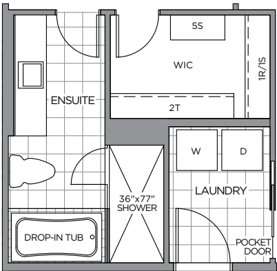
OPTIONAL PRIMARY ENSUITE
