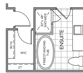
OPT. ENSUITE LAYOUT
